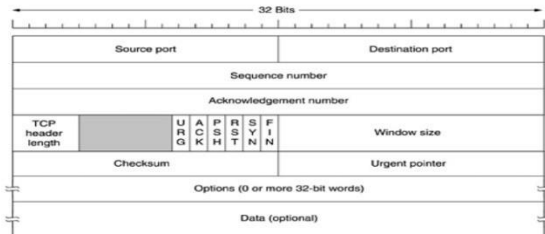
The TCP Header
