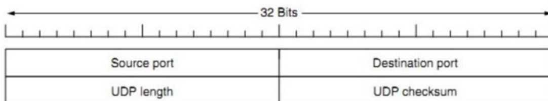
The UDP header
